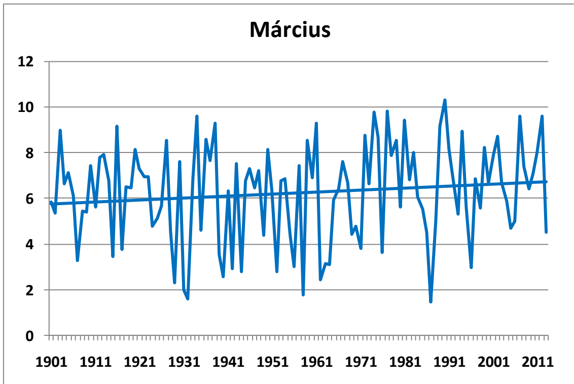
126. ábra. A márciusi középhőmérséklet alakulása 1901-2013 között Budapest történelmi adatsorai alapján (°C), a lineáris trenddel
