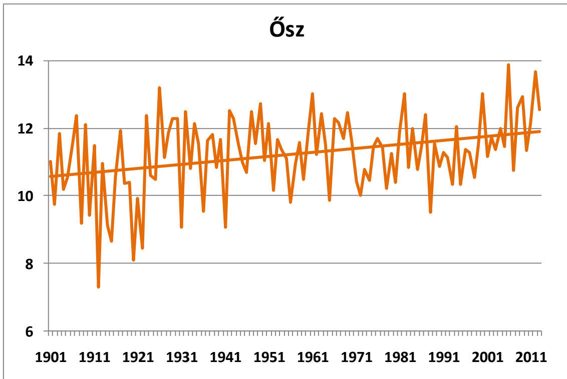
138. ábra. Az őszi középhőmérsékletek alakulása 1901-2013 között Budapest történelmi adatsorai alapján (°C), a lineáris trenddel
