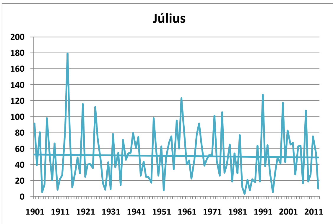
113. ábra. A júliusi csapadékösszegek alakulása 1901-2013 között Budapest történelmi adatai alapján (mm), a lineáris trenddel
