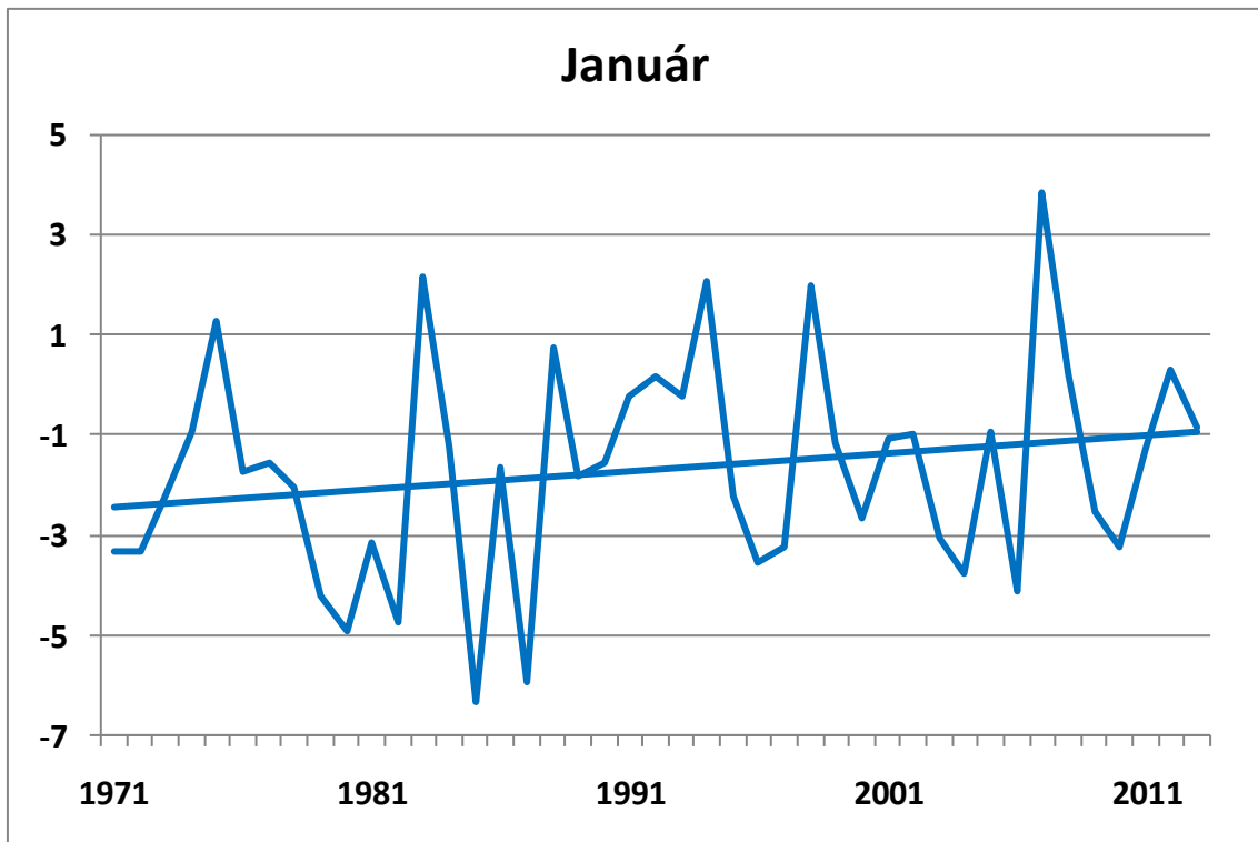
141. ábra. A januári középhőmérsékletek alakulása 1971-2013 között Széchenyi-hegyen (°C), a lineáris trenddel
