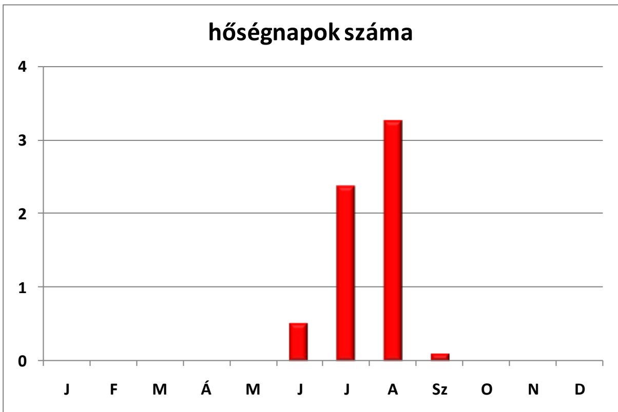
11. ábra. Hőségnapok átlagos száma (1971-2000) Széchenyi-hegy állomás adatai alapján
