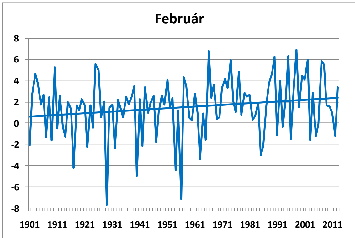
125. ábra. A februári középhőmérsékletek alakulása 1901-2013 között Budapest történelmi adatsorai alapján (°C), a lineáris trenddel
