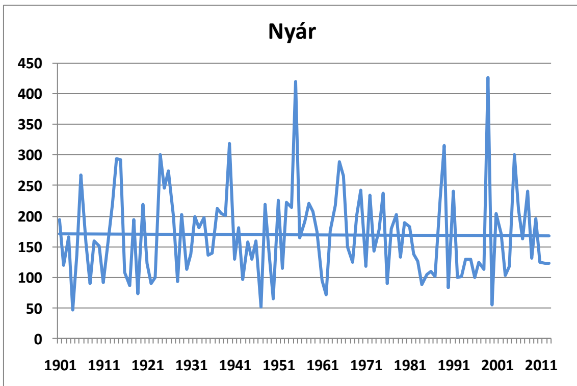
120. ábra. A nyári csapadékösszegek alakulása 1901-2013 között Budapest történelmi adatsorai alapján (mm), a lineáris trenddel
