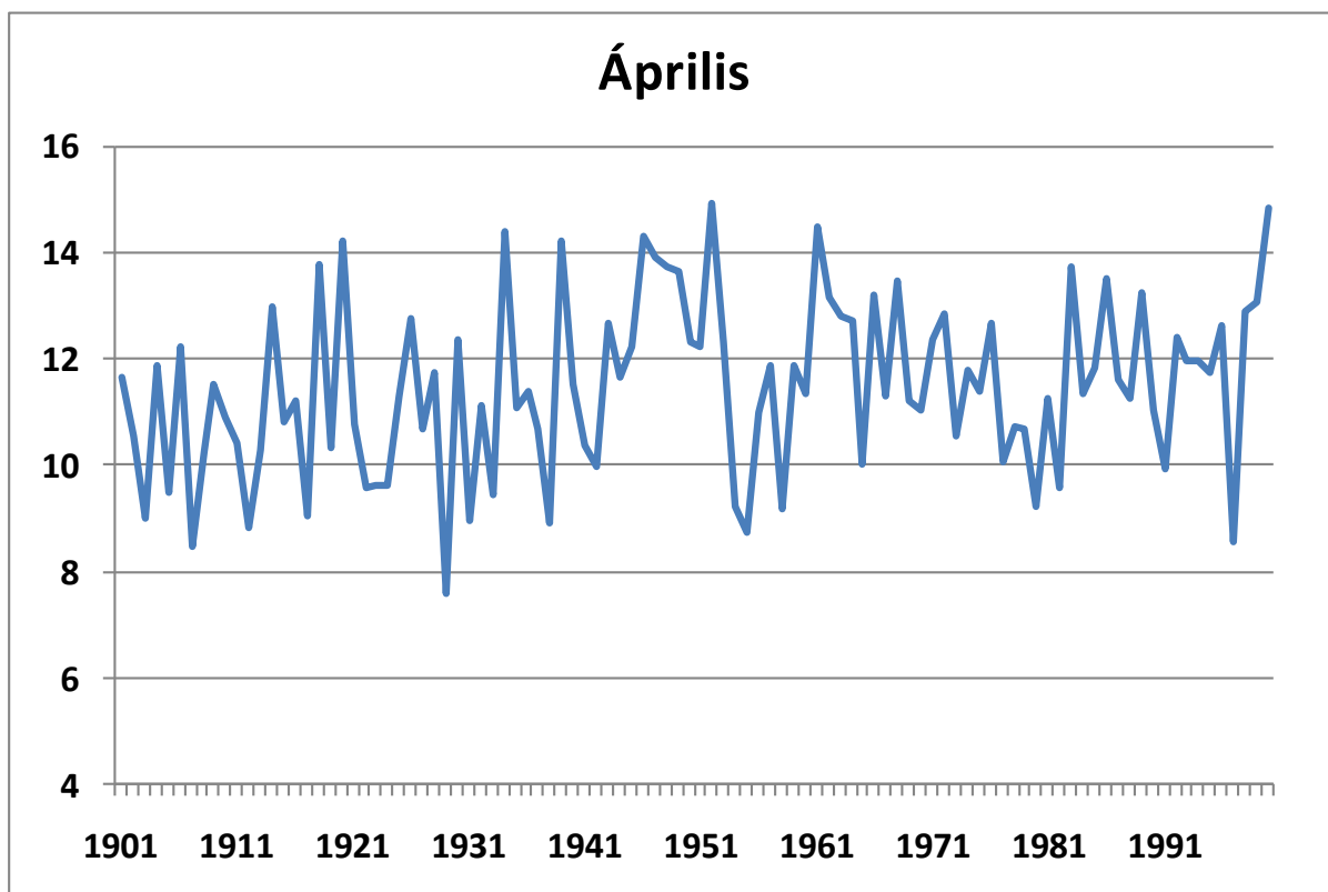
76. ábra. Az áprilisi középhőmérséklet alakulása 1901-2000 között Budapest történelmi adatsorai alapján (°C)
