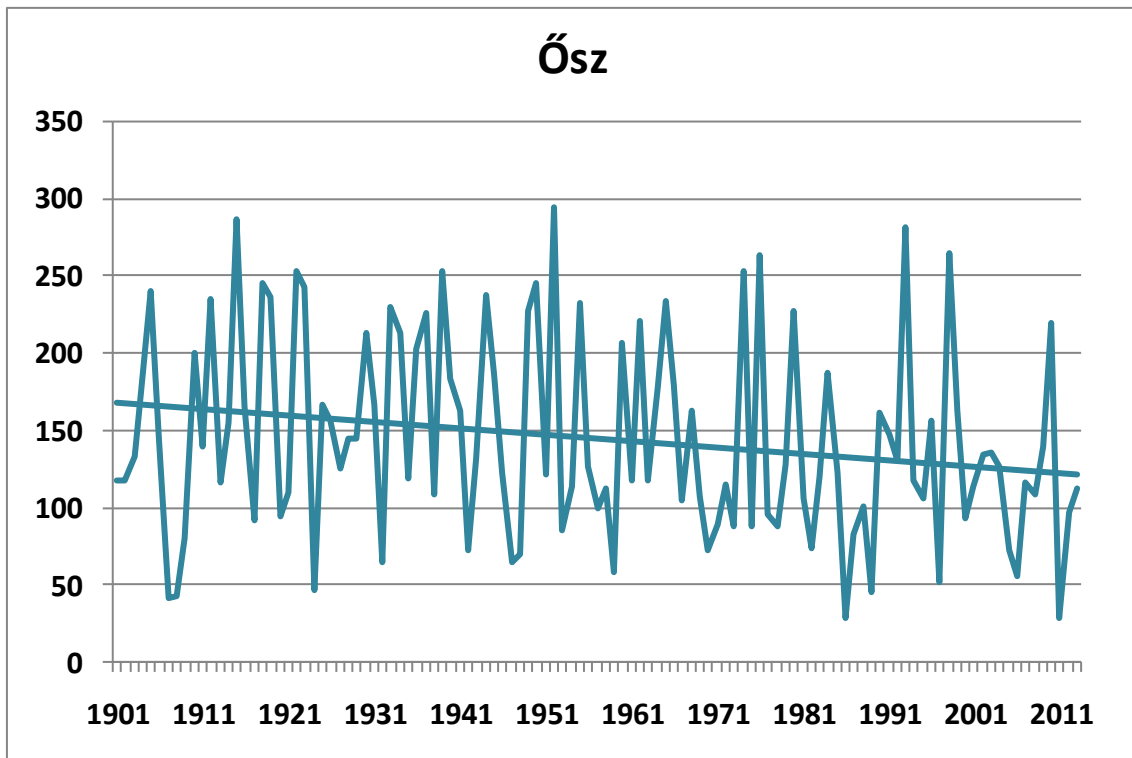
121. ábra. Az őszi csapadékösszegek alakulása 1901-2013 között Budapest történelmi adatsorai alapján (mm), a lineáris trenddel
