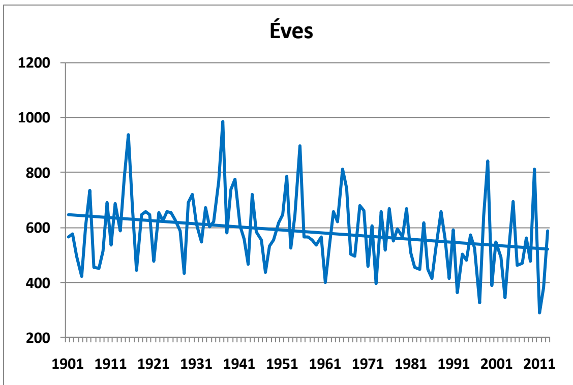
123. ábra. Az éves csapadékösszegek alakulása 1901-2013 között Budapest történelmi adatsorai alapján (mm), a lineáris trenddel
