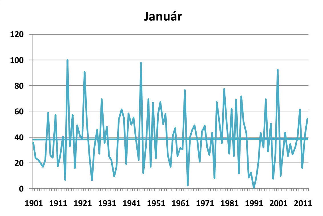
107. ábra. A januári csapadékösszegek alakulása 1901-2013 között Budapest történelmi adatsorai alapján (mm), a lineáris trenddel
