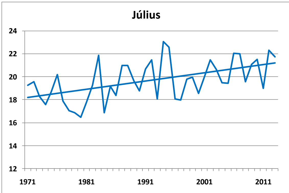
147. ábra. A júliusi középhőmérsékletek alakulása 1971-2013 között Széchenyi-hegyen (°C), a lineáris trenddel
