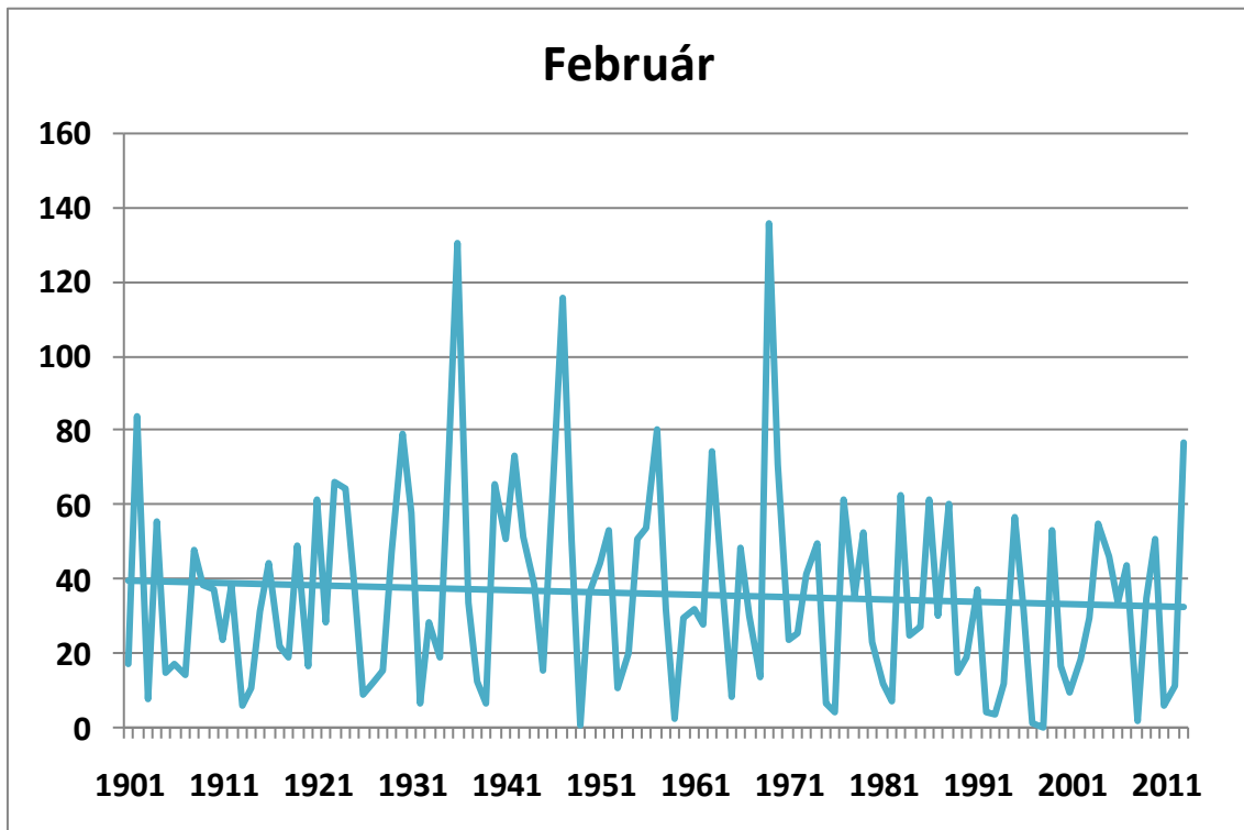
108. ábra. A februári csapadékösszegek alakulása 1901-2013 között Budapest történelmi adatsorai alapján (mm), a lineáris trenddel
