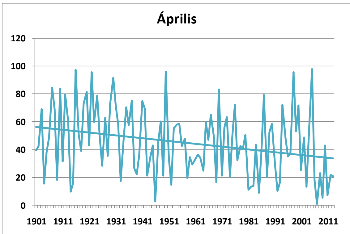
110. ábra. Az áprilisi csapadékösszegek alakulása 1901-2013 között Budapest történelmi adatsorai alapján (mm), a lineáris trenddel
