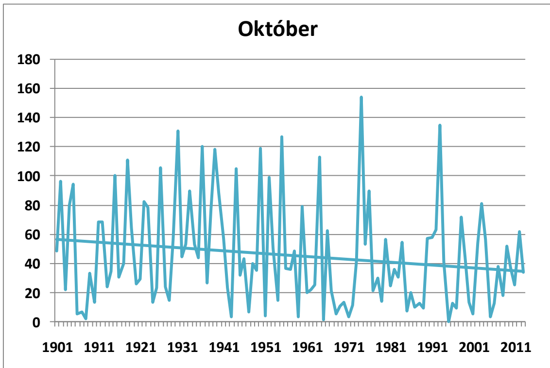
116. ábra. Az októberi csapadékösszegek alakulása 1901-2013 között Budapest történelmi adatsorai alapján (mm), a lineáris trenddel
