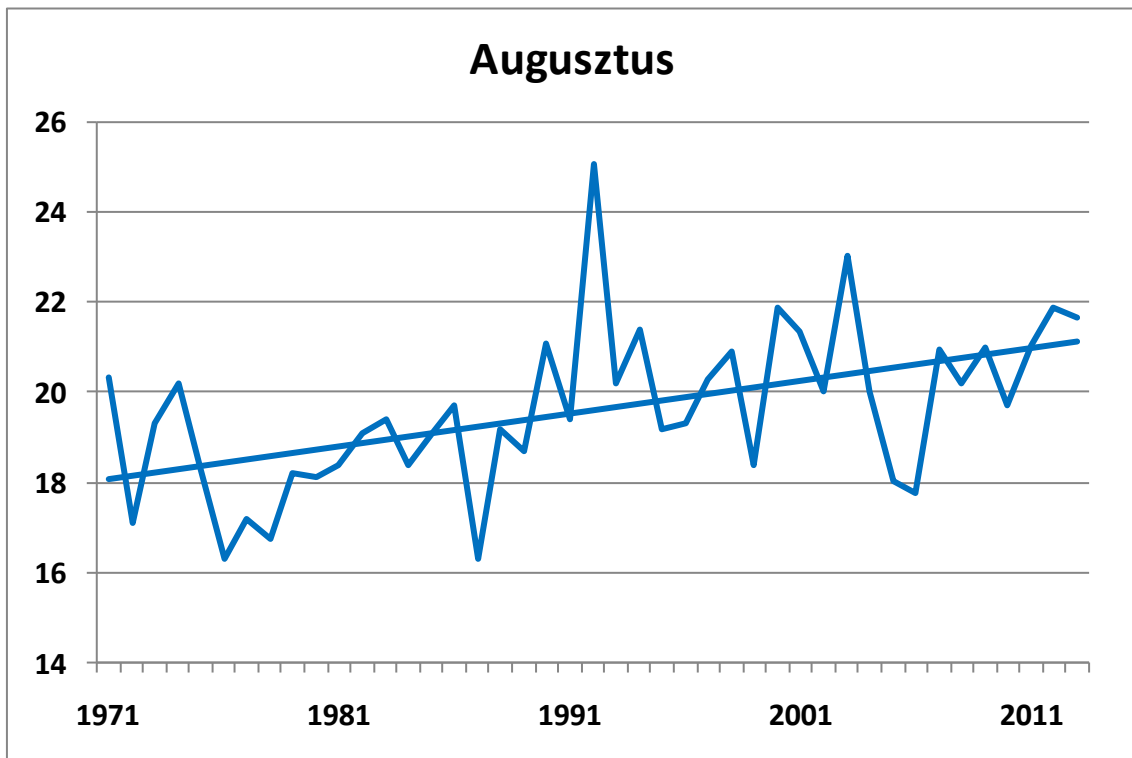
148. ábra. Az augusztusi középhőmérsékletek alakulása 1971-2013 között Széchenyi-hegyen (°C), a lineáris trenddel
