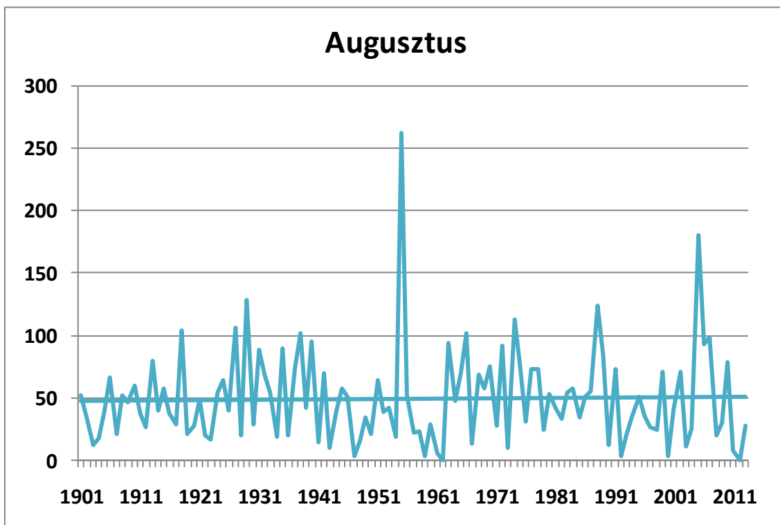
114. ábra. Az augusztusi csapadékösszegek alakulása 1901-2013 között Budapest történelmi adatai alapján (mm), a lineáris trenddel
