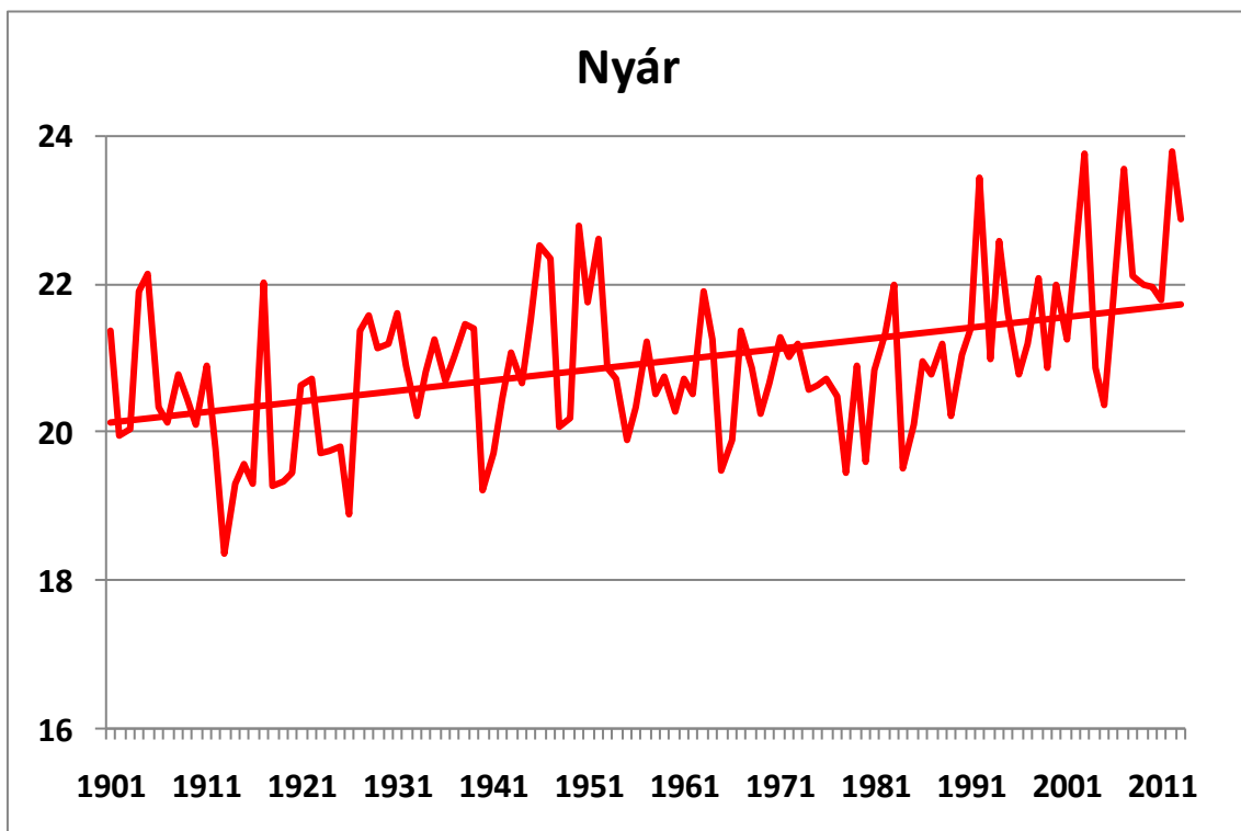
137. ábra. A nyári középhőmérsékletek alakulása 1901-2013 között Budapest történelmi adatsorai alapján (°C), a lineáris trenddel
