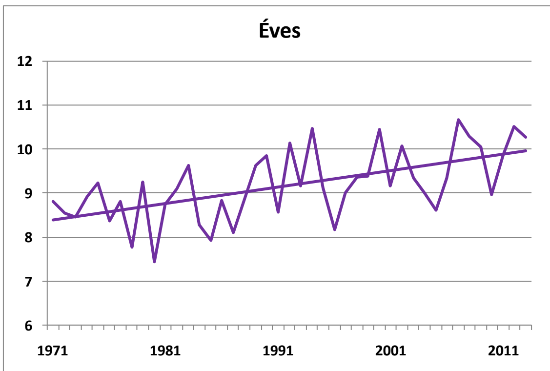
157. ábra. Az éves középhőmérsékletek alakulása 1971-2013 között Széchenyi-hegyen (°C), a lineáris trenddel
