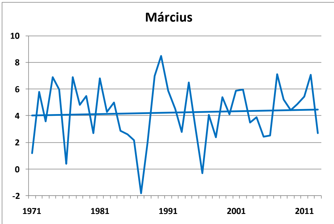
143. ábra. A márciusi középhőmérsékletek alakulása 1971-2013 között Széchenyi-hegyen (°C), a lineáris trenddel
