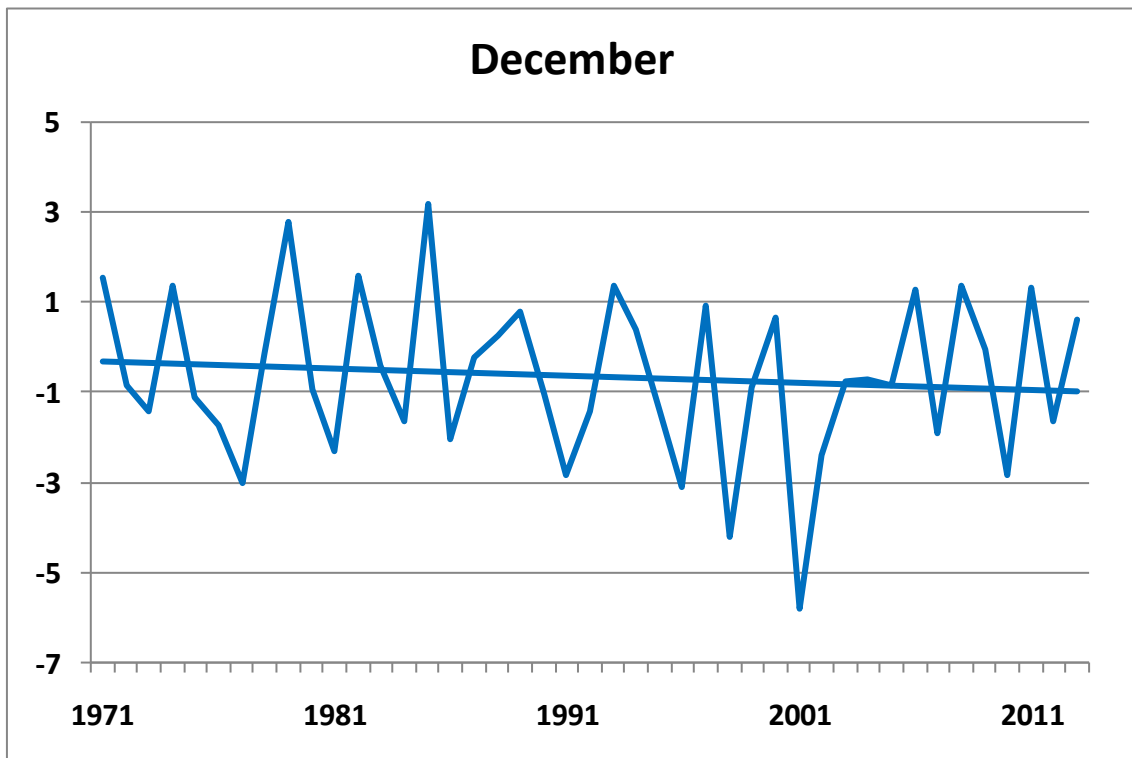
152. ábra. A decemberi középhőmérsékletek alakulása 1971-2013 között Széchenyi-hegyen (°C), a lineáris trenddel
