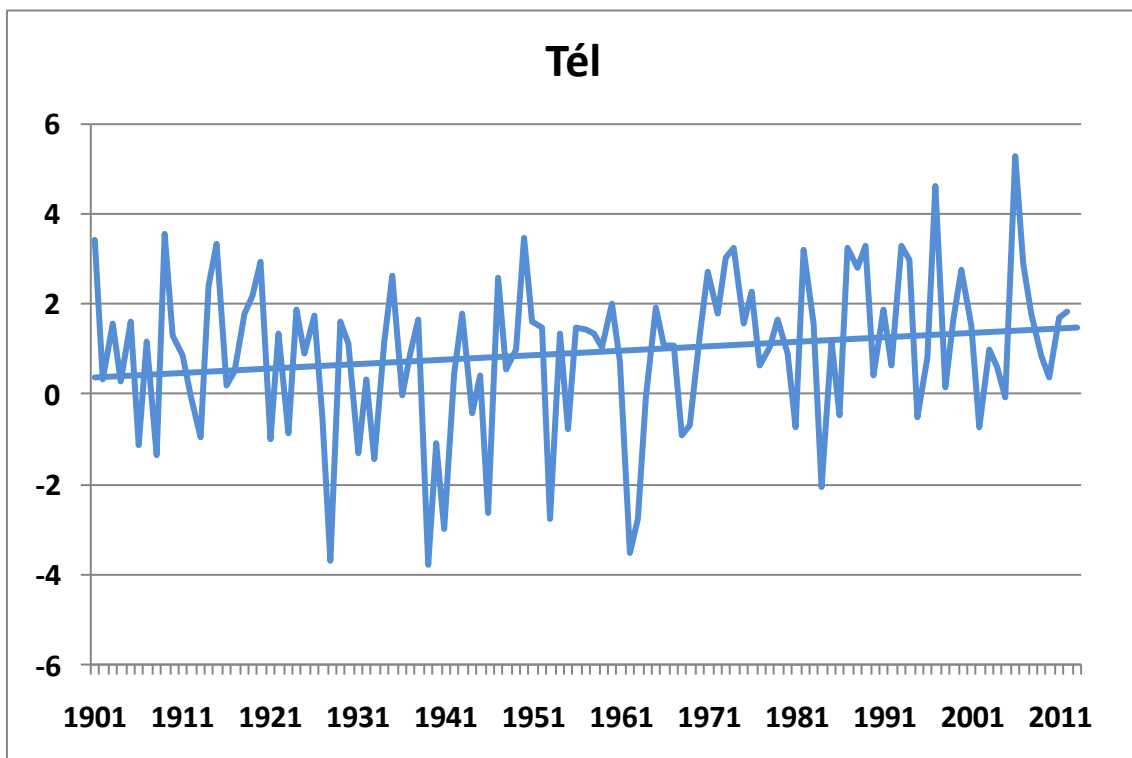
139. ábra. A téli középhőmérsékletek alakulása 1901-2013 között Budapest történelmi adatsorai alapján (°C), a lineáris trenddel
