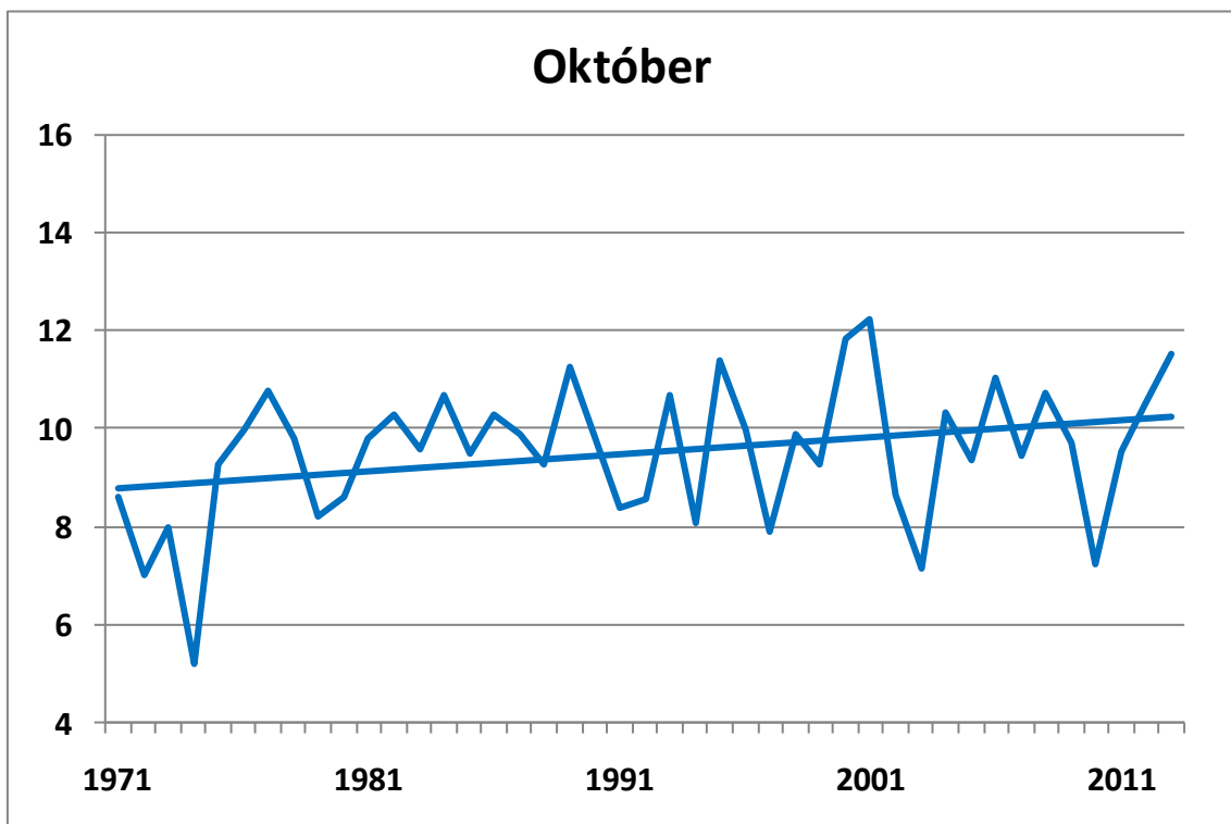
150. ábra. Az októberi középhőmérsékletek alakulása 1971-2013 között Széchenyi-hegyen (°C), a lineáris trenddel
