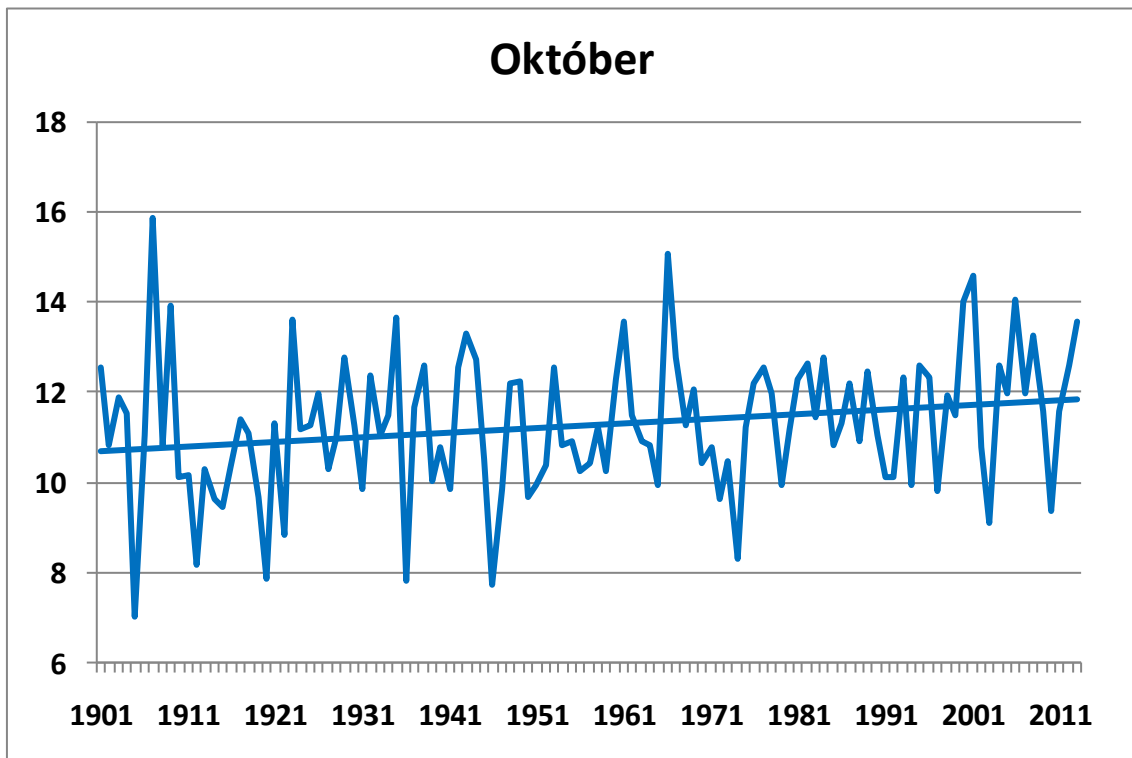
133. ábra. Az októberi középhőmérsékletek alakulása 1901-2013 között Budapest történelmi adatsorai alapján (°C), a lineáris trenddel
