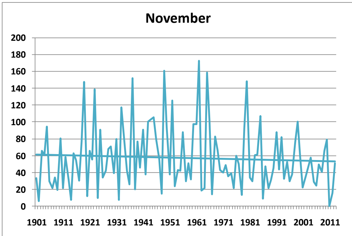
117. ábra. A novemberi csapadékösszegek alakulása 1901-2013 között Budapest történelmi adatsorai alapján (mm), a lineáris trenddel
