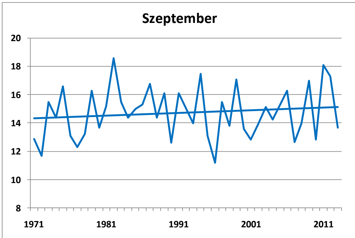
149. ábra. A szeptemberi középhőmérsékletek alakulása 1971-2013 között Széchenyi-hegyen (°C), a lineáris trenddel
