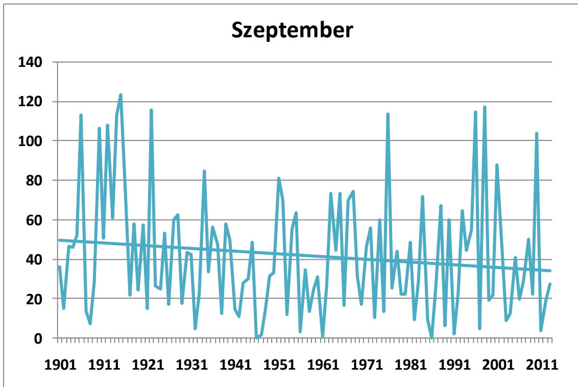
115. ábra. A szeptemberi csapadékösszegek alakulása 1901-2013 között Budapest történelmi adatsorai alapján (mm), a lineáris trenddel
