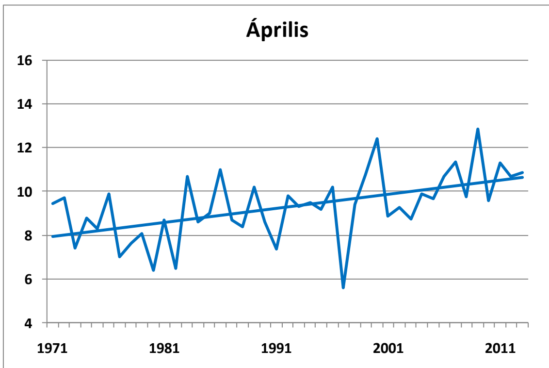
144. ábra. Az áprilisi középhőmérsékletek alakulása 1971-2013 között Széchenyi-hegyen (°C), a lineáris trenddel
