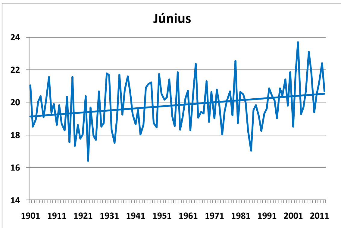
129. ábra. A júniusi középhőmérsékletek alakulása 1901-2013 között Budapest történelmi adatsorai alapján (°C), a lineáris trenddel
