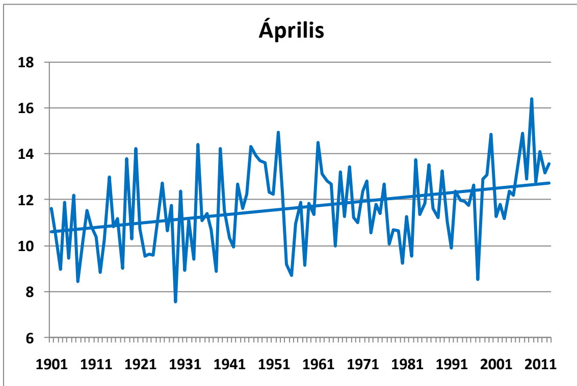
127. ábra. Az áprilisi középhőmérséklet alakulása 1901-2013 között Budapest történelmi adatsorai alapján (°C), a lineáris trenddel
