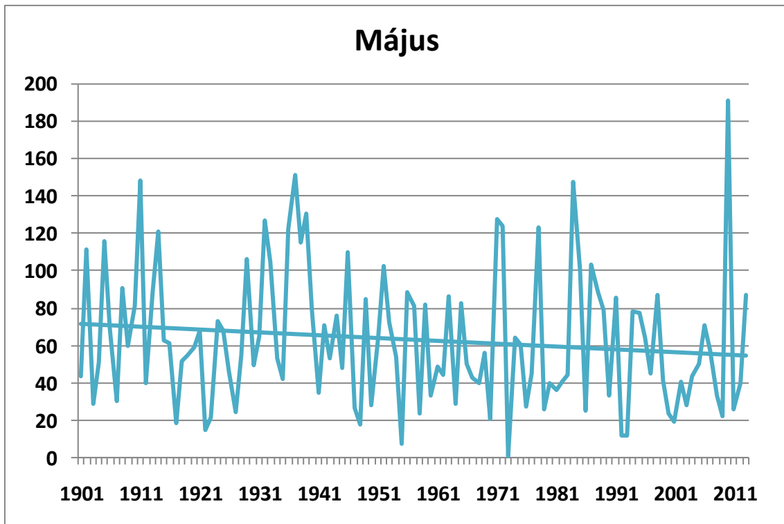
111. ábra. A májusi csapadékösszegek alakulása 1901-2013 között Budapest történelmi adatsorai alapján (mm), a lineáris trenddel
