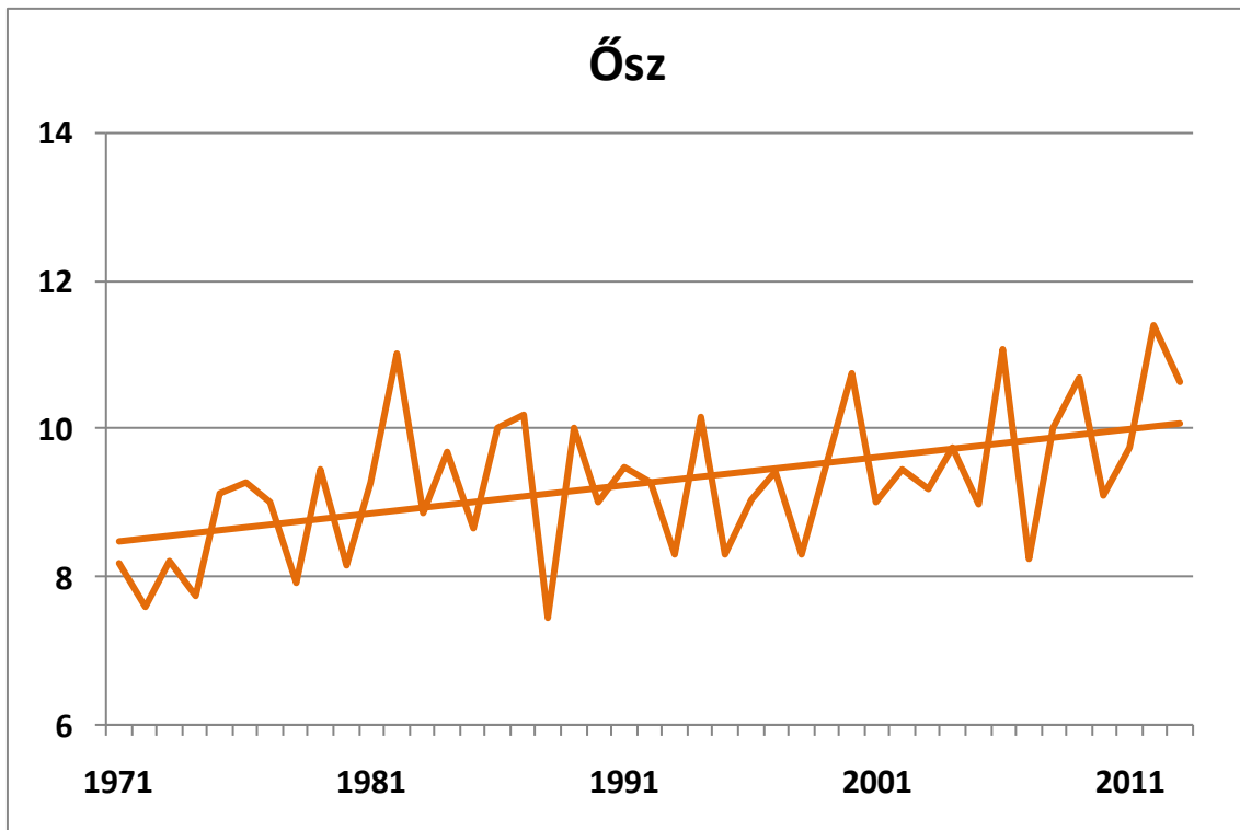
155. ábra. Az őszi középhőmérsékletek alakulása 1971-2013 között Széchenyi-hegyen (°C), a lineáris trenddel
