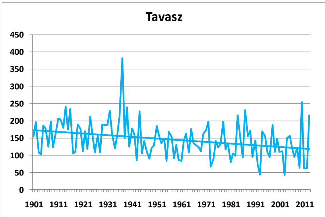
119. ábra. A tavaszi csapadékösszegek alakulása 1901-2013 között Budapest történelmi adatsorai alapján (mm), a lineáris trenddel
