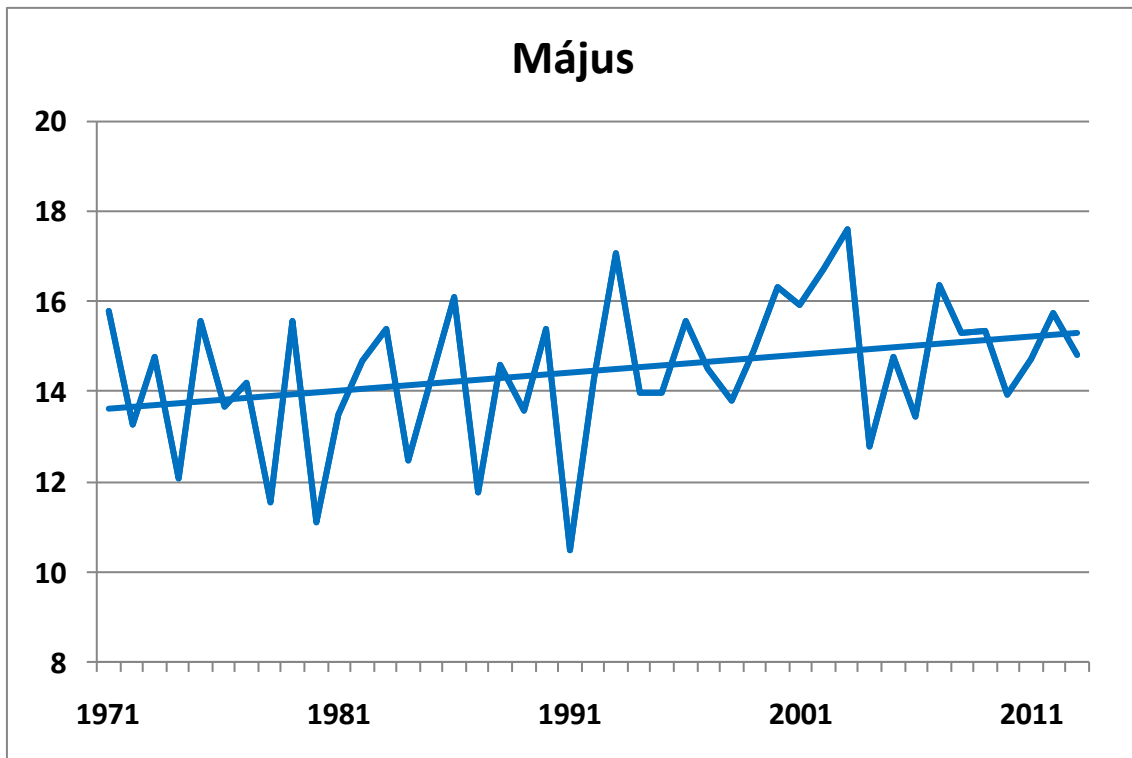
145. ábra. A májusi középhőmérsékletek alakulása 1971-2013 között Széchenyi-hegyen (°C), a lineáris trenddel
