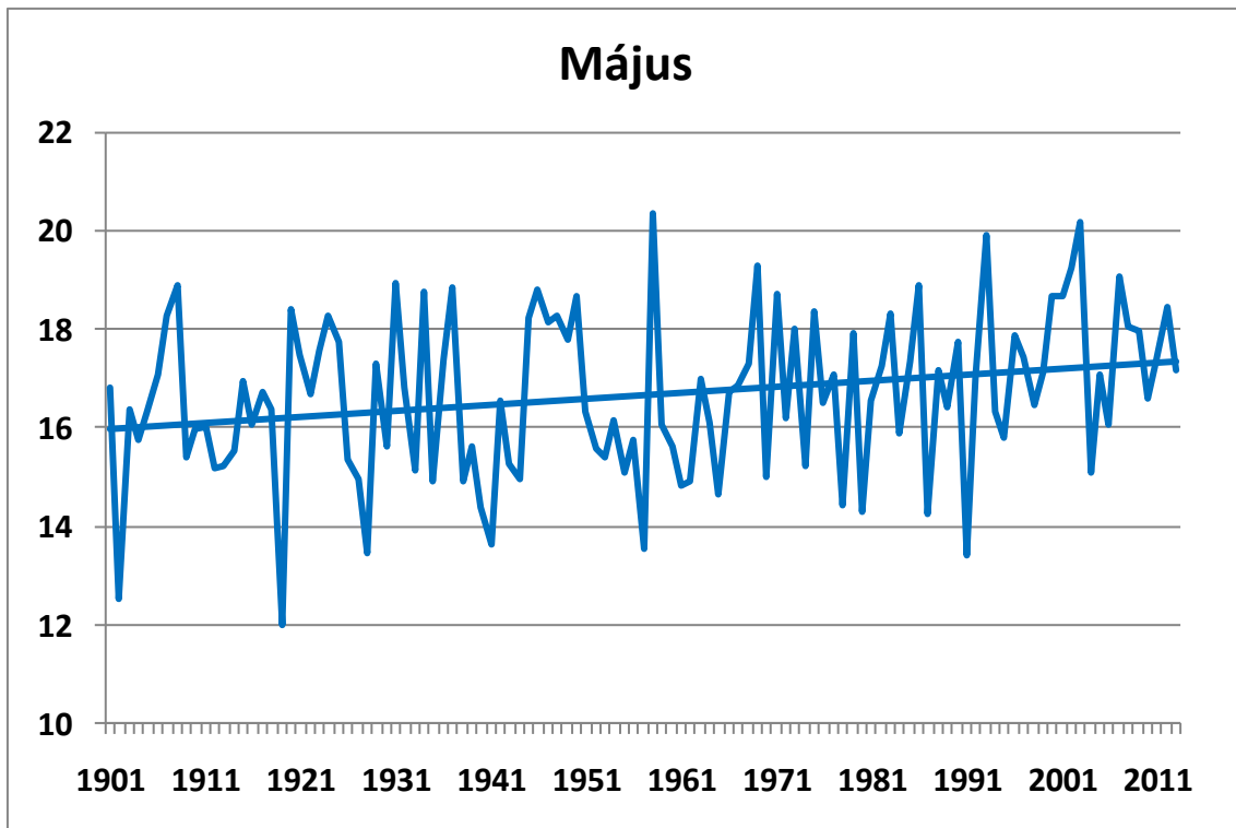
128. ábra. A májusi középhőmérsékletek alakulása 1901-2013 között Budapest történelmi adatsorai alapján (°C), a lineáris trenddel
