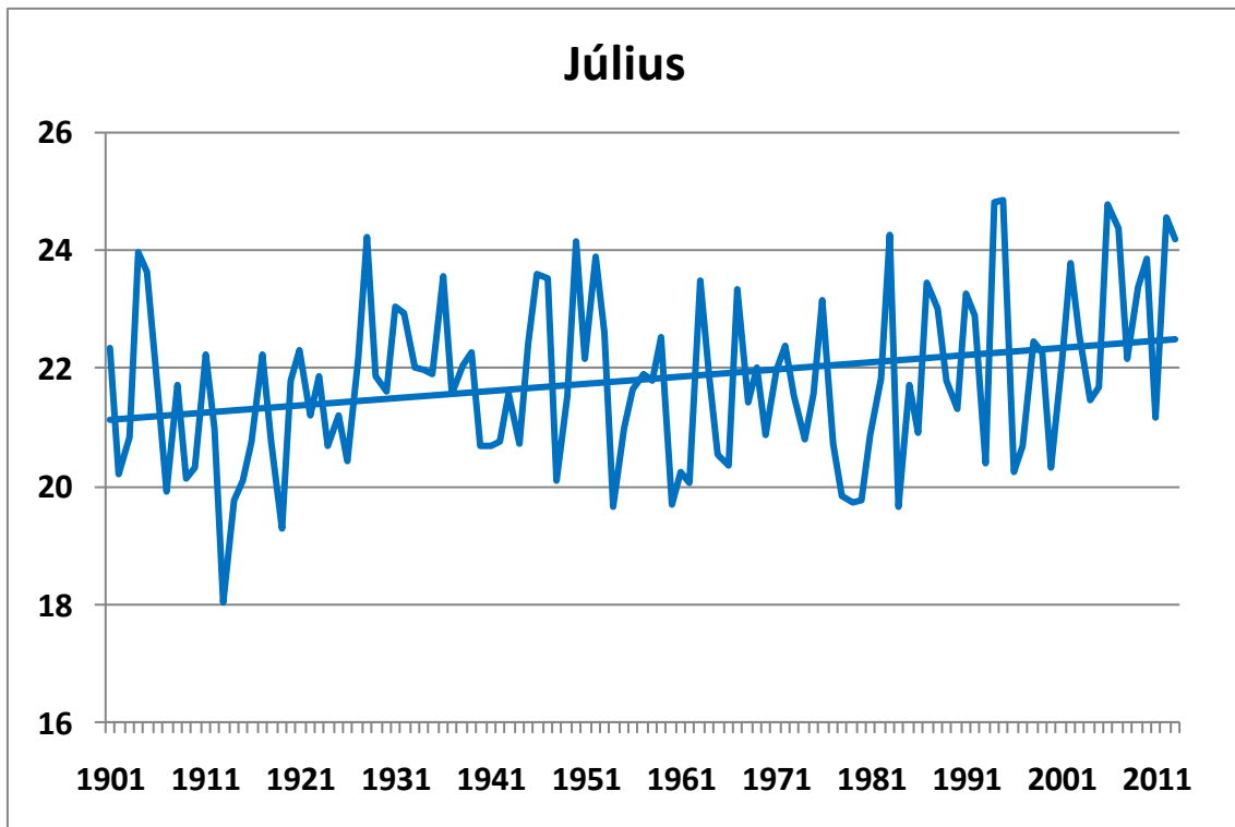
130. ábra. A júliusi középhőmérsékletek alakulása 1901-2013 között Budapest történelmi adatsorai alapján (°C), a lineáris trenddel
