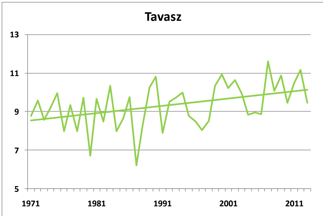
153. ábra. A tavaszi középhőmérséklet alakulása 1971-2013 között Széchenyi-hegyen (°C), a lineáris trenddel
