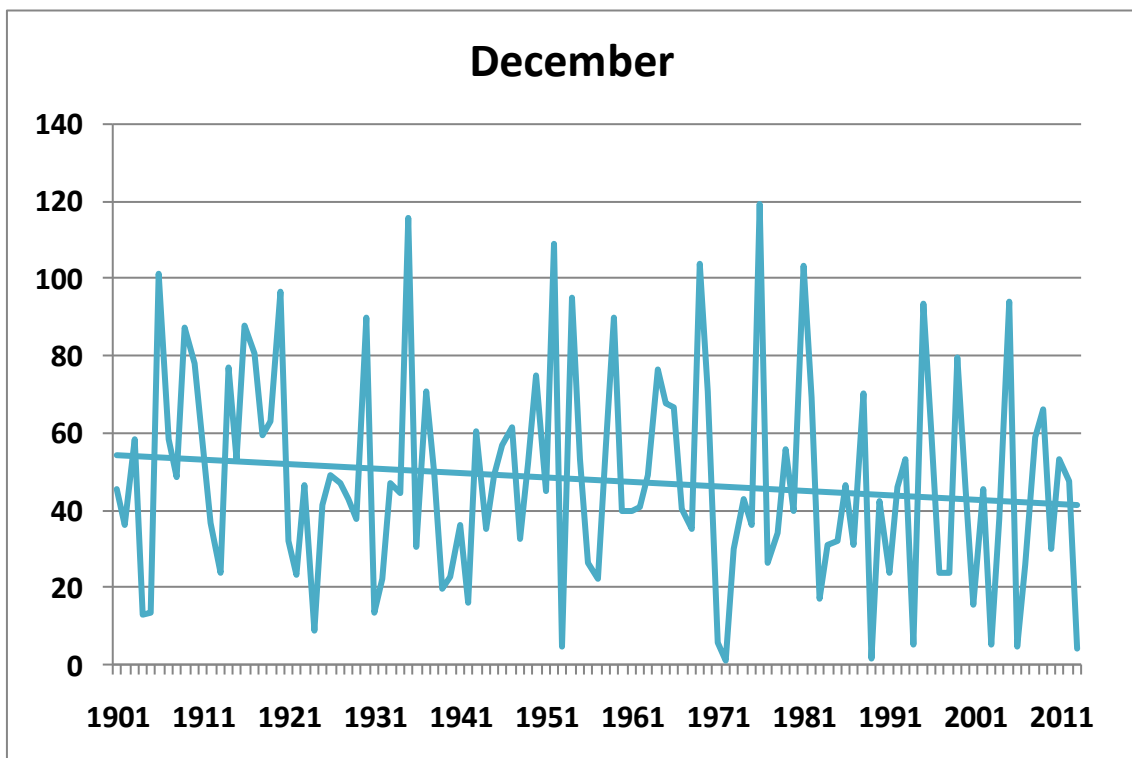
118. ábra. A decemberi csapadékösszegek alakulása 1901-2013 között Budapest történelmi adatsorai alapján (mm), a lineáris trenddel
