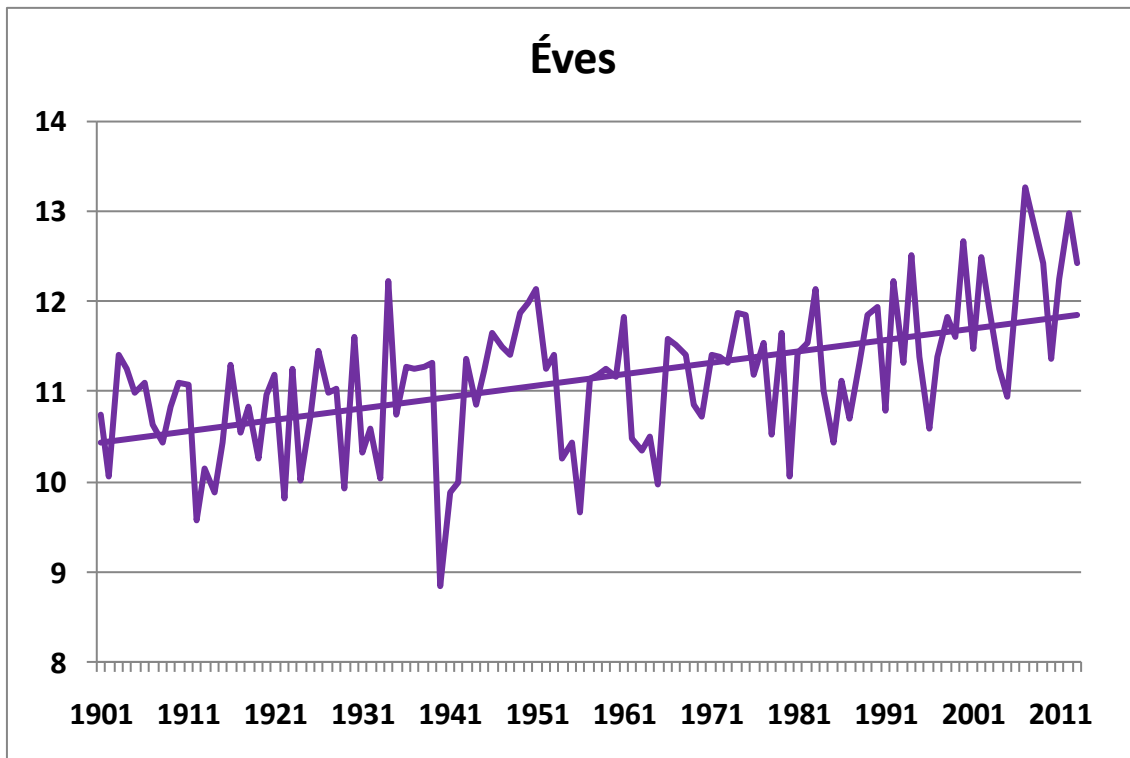
140. ábra. Az éves középhőmérsékletek alakulása 1901-2013 között Budapest történelmi adatsorai alapján (°C), a lineáris trenddel
