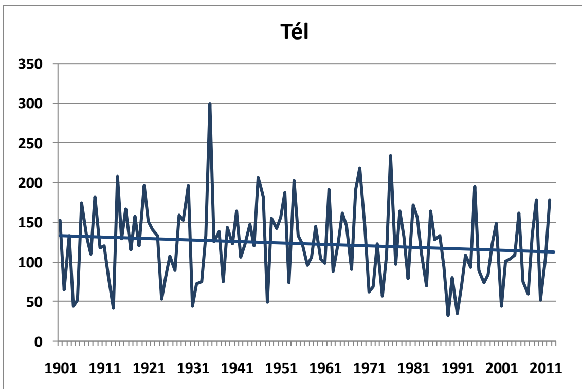
122. ábra. A téli csapadékösszegek alakulása 1901-2013 között Budapest történelmi adatsorai alapján (mm), a lineáris trenddel
