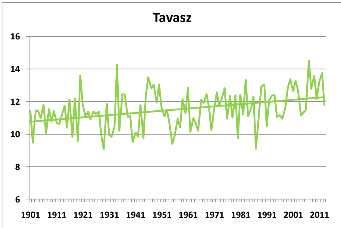
136. ábra. A tavaszi középhőmérsékletek alakulása 1901-2013 között Budapest történelmi adatsorai alapján (°C), a lineáris trenddel
