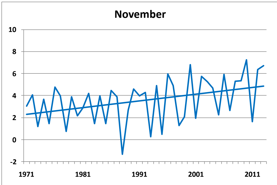
151. ábra. A novemberi középhőmérsékletek alakulása 1971-2013 között Széchenyi-hegyen (°C), a lineáris trenddel
