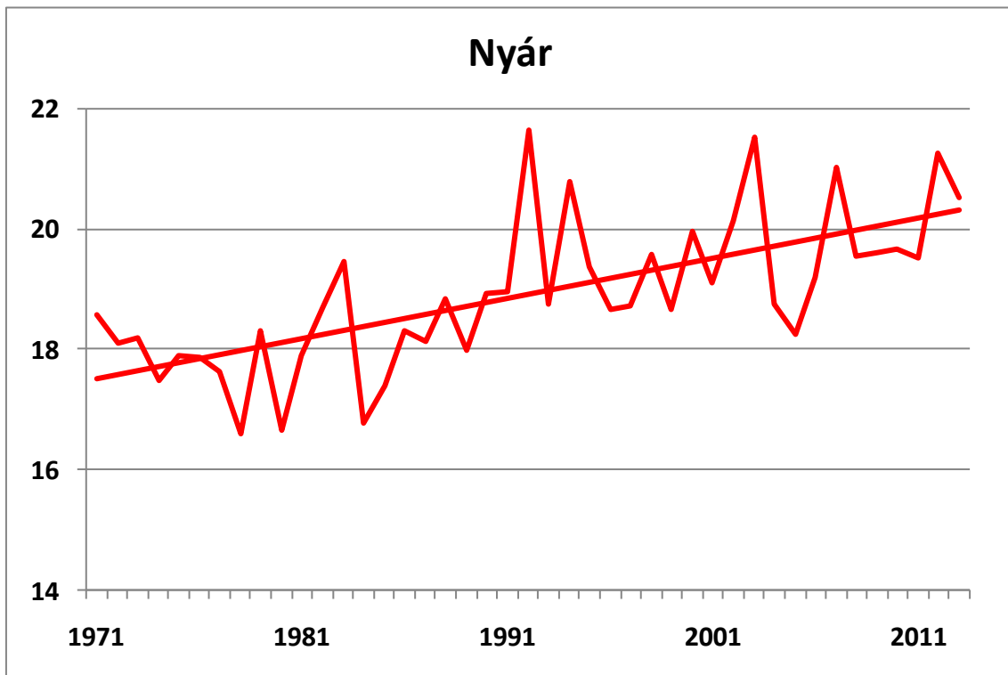
154. ábra. A nyári középhőmérséklet alakulása 1971-2013 között Széchenyi-hegyen (°C), a lineáris trenddel
