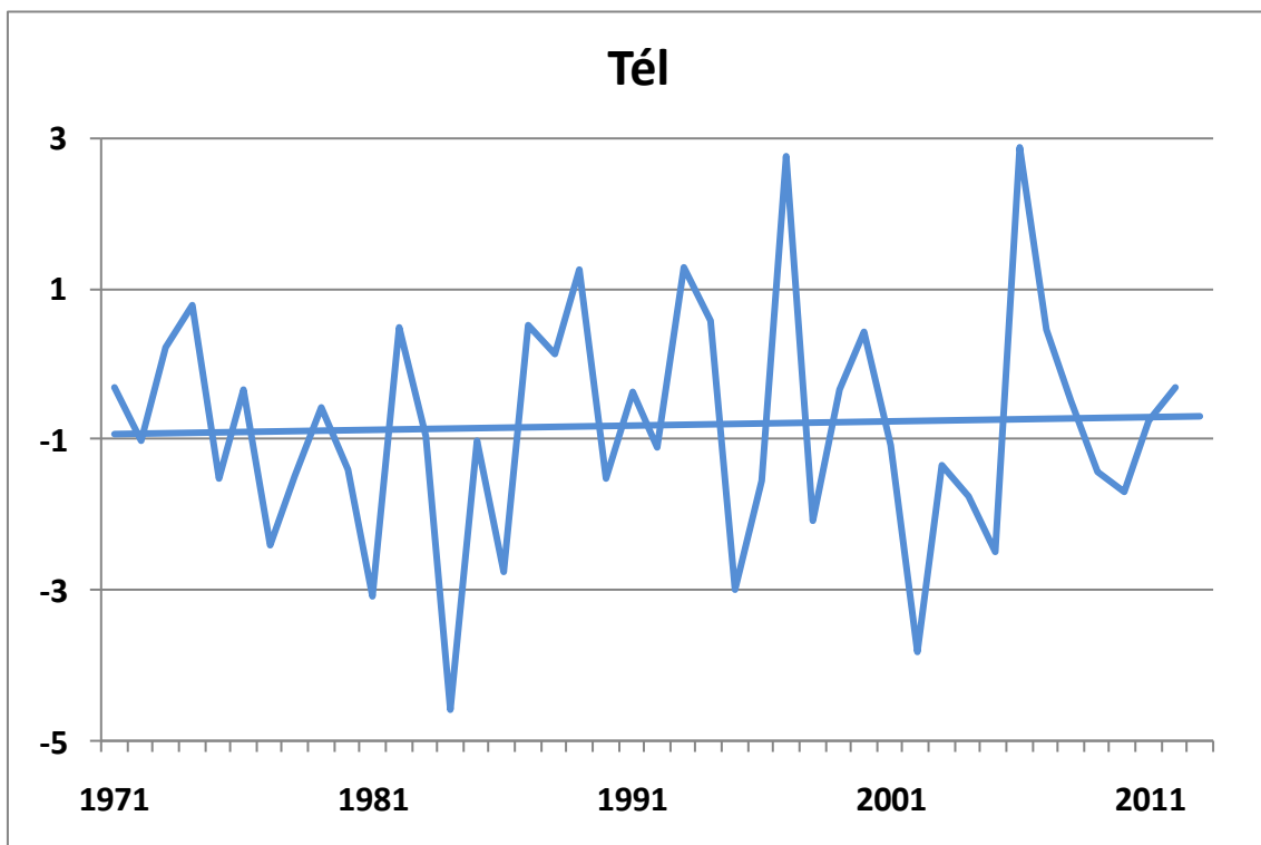
156. ábra. A téli középhőmérsékletek alakulása 1971-2013 között Széchenyi-hegyen (°C), a lineáris trenddel
