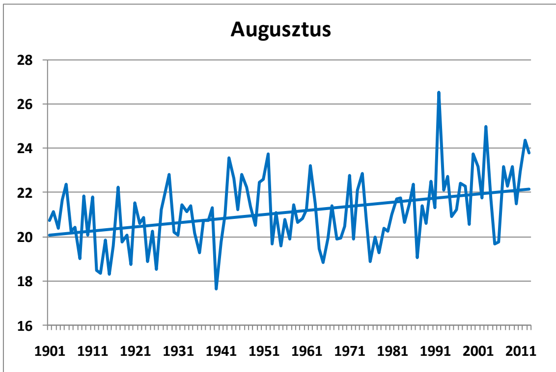
131. ábra. Az augusztusi középhőmérsékletek alakulása 1901-2013 között Budapest történelmi adatsorai alapján (°C), a lineáris trenddel
