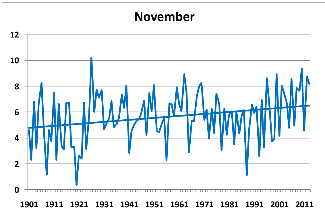
134. ábra. A novemberi középhőmérsékletek alakulása 1901-2013 között Budapest történelmi adatsorai alapján (°C), a lineáris trenddel
