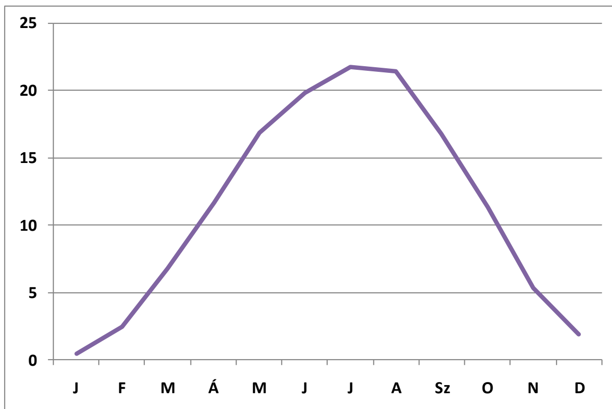
2. ábra. Havi középhőmérsékletek sokéves (1971-2000) átlaga, Budapest, Kitaibel Pál utca (°C)
