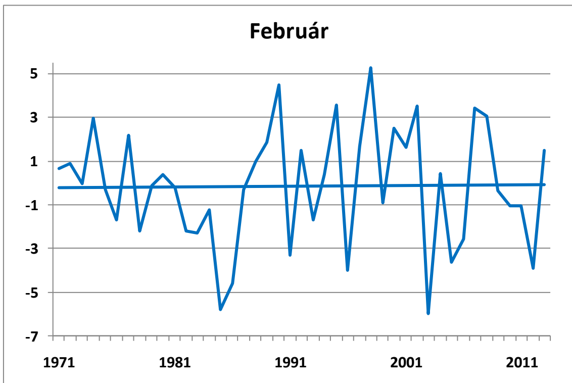
142. ábra. A februári középhőmérsékletek alakulása 1971-2013 között Széchenyi-hegyen (°C), a lineáris trenddel
