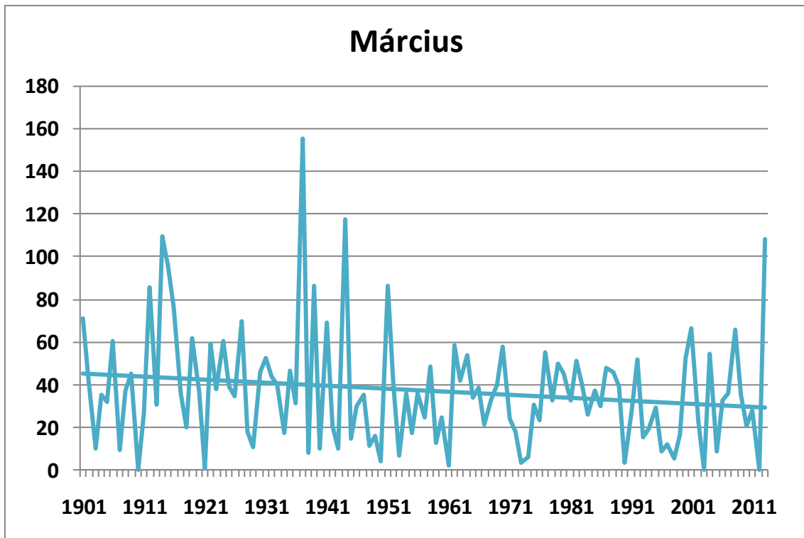
109. ábra. A márciusi csapadékösszegek alakulása 1901-2013 között Budapest történelmi adatsorai alapján (mm), a lineáris trenddel
