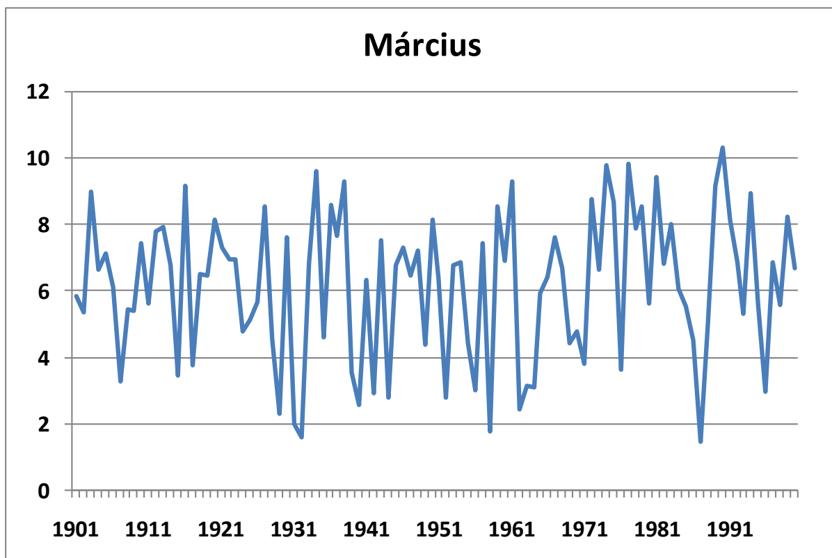
75. ábra. A márciusi középhőmérséklet alakulása 1901-2000 között Budapest történelmi adatsorai alapján (°C)
