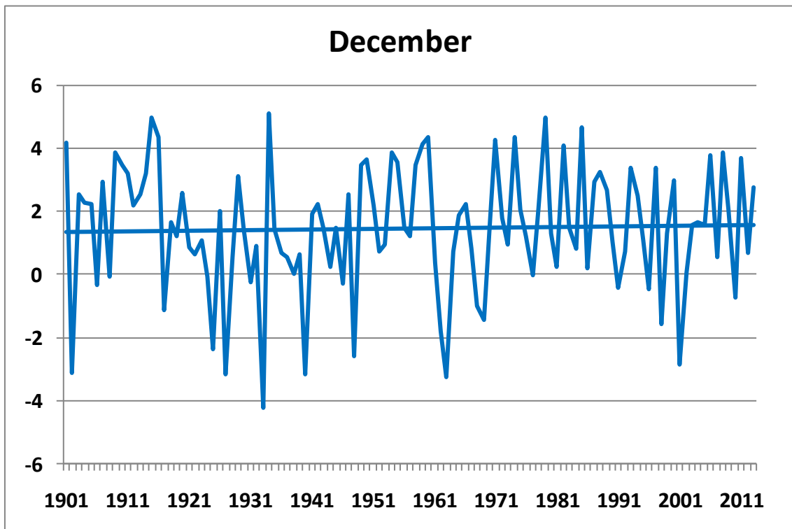
135. ábra. A decemberi középhőmérsékletek alakulása 1901-2013 között Budapest történelmi adatsorai alapján (°C), a lineáris trenddel
