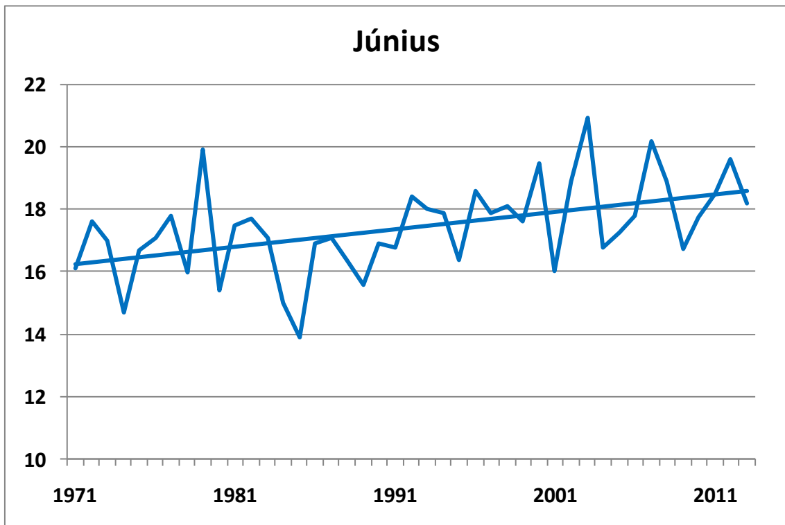
146. ábra. A júniusi középhőmérsékletek alakulása 1971-2013 között Széchenyi-hegyen (°C), a lineáris trenddel
