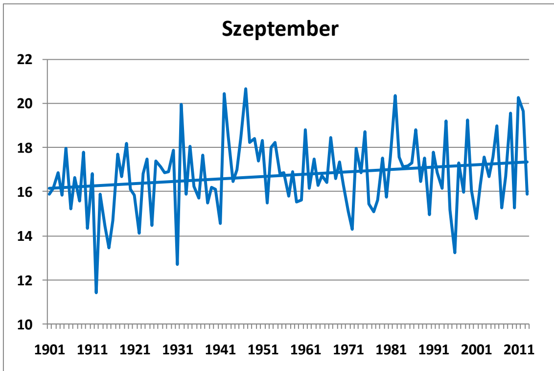
132. ábra. A szeptemberi középhőmérsékletek alakulása 1901-2013 között Budapest történelmi adatsorai alapján (°C), a lineáris trenddel
