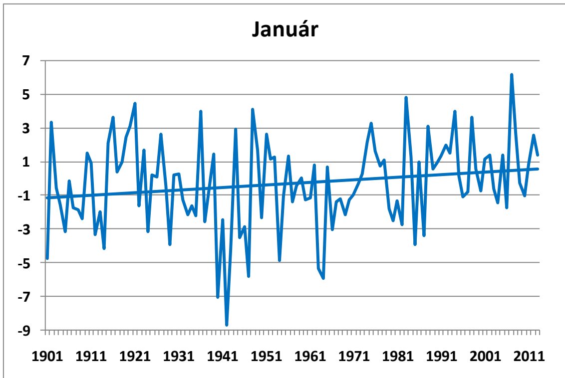
124. ábra. A januári középhőmérsékletek alakulása 1901-2013 között Budapest történelmi adatsorai alapján (°C), a lineáris trenddel
