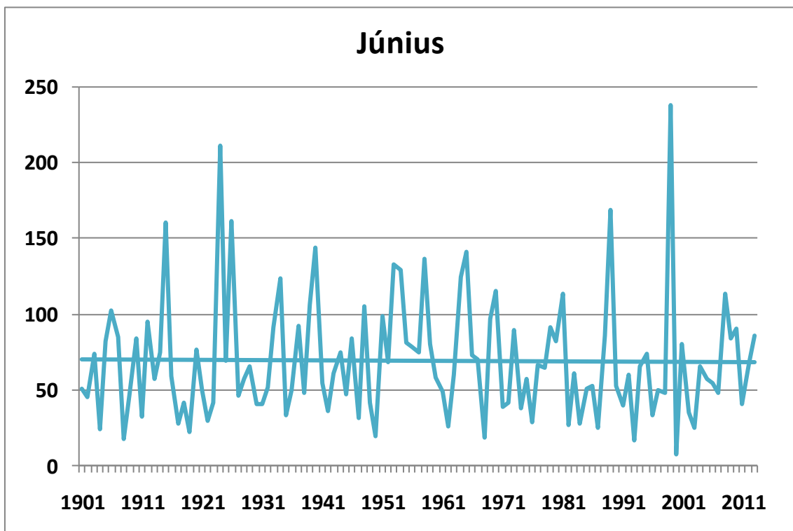
112. ábra. A júniusi csapadékösszegek alakulása 1901-2013 között Budapest történelmi adatsorai alapján (mm), a lineáris trenddel
