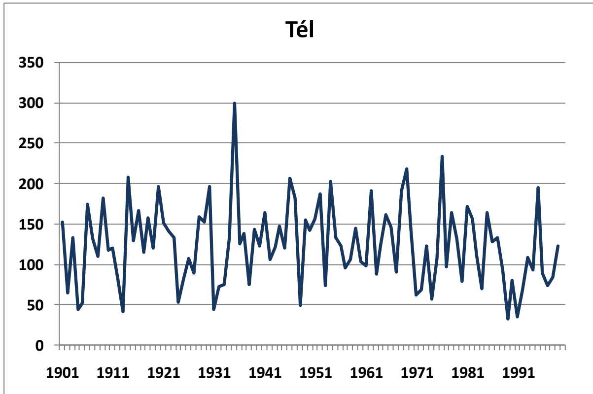
105. ábra. A téli csapadékösszegek alakulása 1901-2000 között Budapest történelmi adatsorai alapján (mm)
